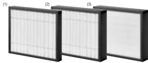
(1) Vorfilter Außenluft ePM10 50% (M5) (2) Abluftfilter ePM10 50% (M5) (3) Außen- o. Abluftfilter ePM1 55% (F7) Außenluftfilter ePM1 80% (F9)
